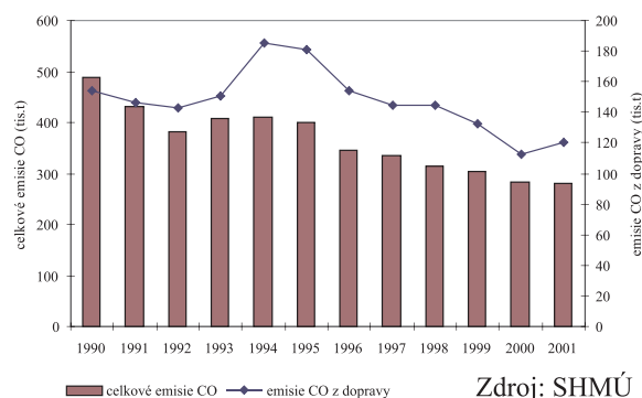
Graf 181. Vývoj emisií CO z dopravnej prevádzky v porovnaní s celkovými emisiami CO
