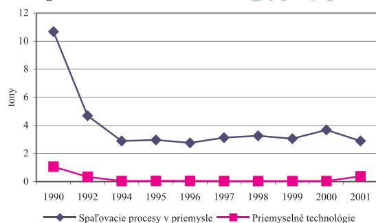
Graf 131. Hg
