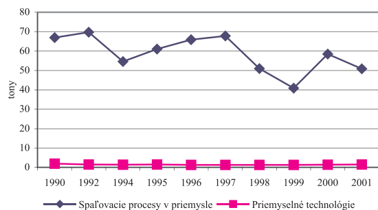
Graf 129. Pb
