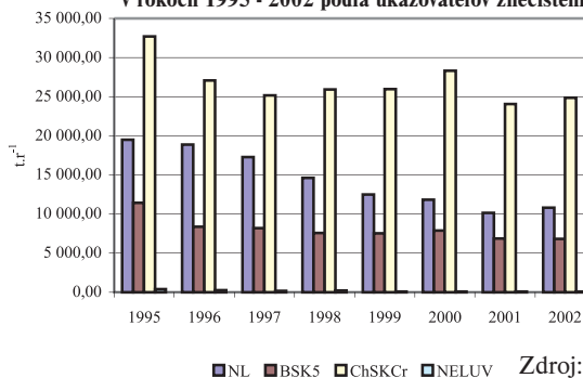
Graf 150. Vypúšťané znečistenie priemyselných odpadových vôd v rokoch 1995 - 2002 podľa ukazovateľov znečistenia (t.r -1 )
