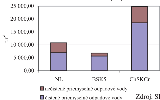
Graf 149. Vypúšťané znečistenie priemyselných odpadových vôd podľa ukazovateľov znečistenia v roku 2002 (t.r -1 )
