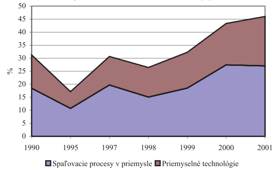
Graf 144. Podiel priemyselných procesov na celkových emisiách PCDD/PCDF* v rokoch 1990 - 2001 (%)
