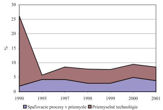
Graf 148. Podiel priemyslu na celkových emisiách PAH v rokoch 1990 - 2001 (%)
