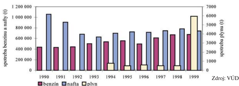
Graf č. 163: Vývoj celkovej spotreby palív v cestnej doprave
