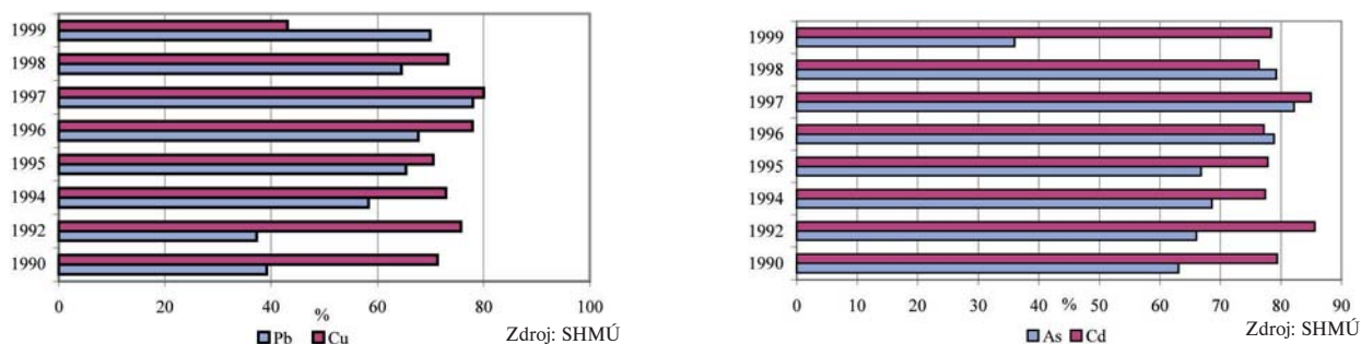
Graf č. 102: Podiel termických priemyselných odvetví na celkových emisiách ťažkých kovov v rokoch 1990 - 1999 (v%)
