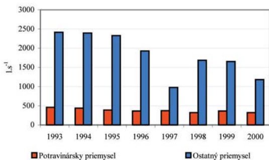
Graf č. 96: Spotreba podzemnej vody v priemysle
