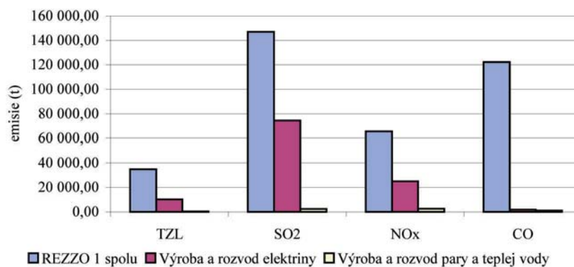
Graf č. 126: Podiel emisií z energetiky na celkových emisiách ZZZ zdrojov REZZO 1 v roku 1999
